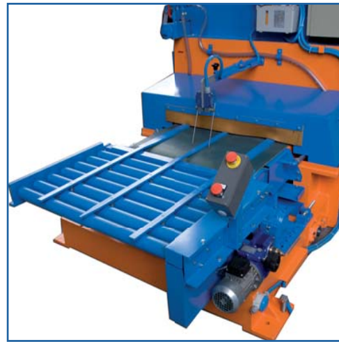
Driven roller, grinder loading. Rodillos motorizados entrada a pulidora.
