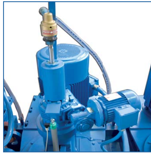
Upward/ descent motor reducer / abrasive working pressure, rotating joint water feeding, abrasive position of sensor. Motorreductor subida/bajada/presión de trabajo del abrasivo, junta rotante alimentación agua, sensor posición abrasivo.
