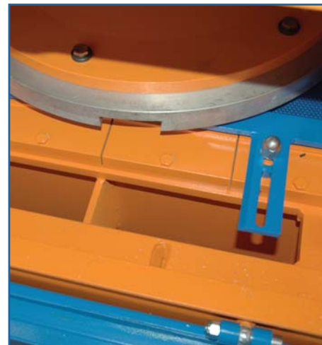
Unloads for grinding water and mud of big dimensions and easy cleaning. Descarga de agua y lodo del pulido de grandes dimensiones y fácil limpieza.
