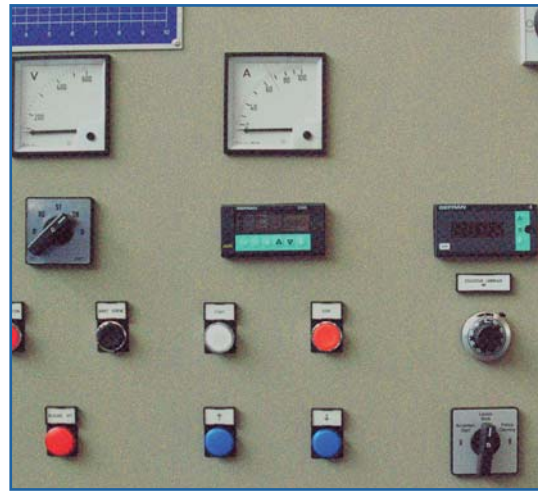
Upward/ descent control of diamond tool and level visualizer. Control subida/bajada del utensilio diamantado y visualizador de cuota.
